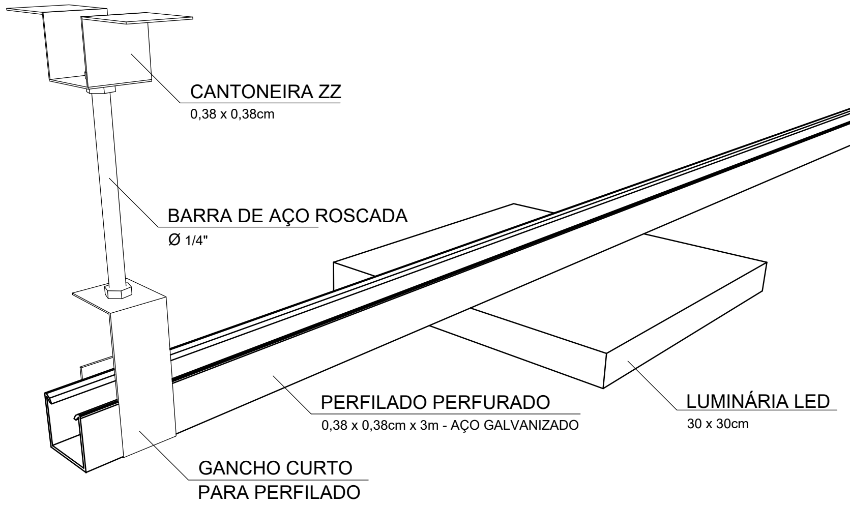
4 DETALHE DE FIXAÇÃO DAS LUMINÁRIAS EM PERFILADOS S/ESC.
