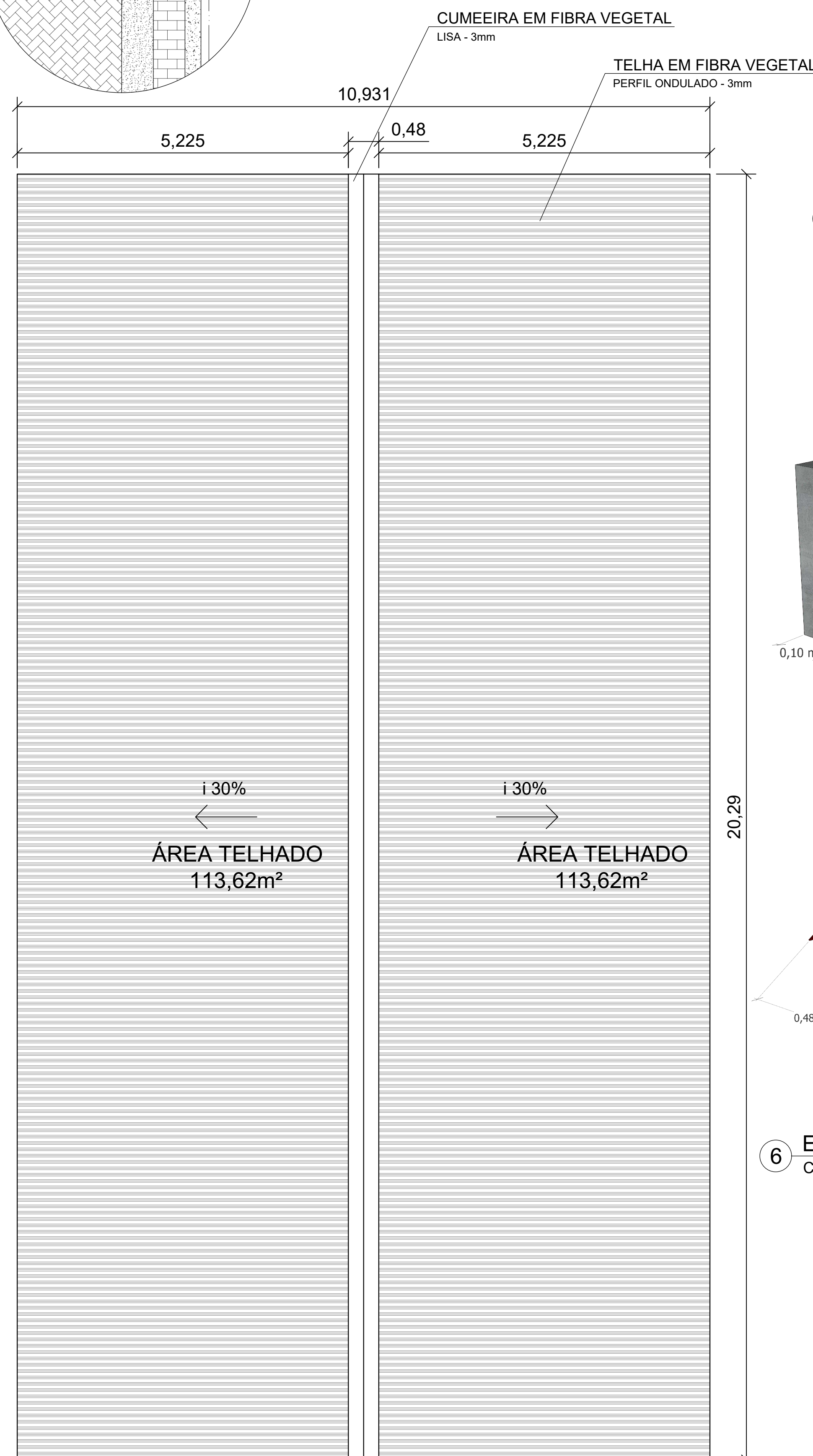
2 PLANTA DE COBERTURA INCLINAÇÃO - ESC. 1:50
