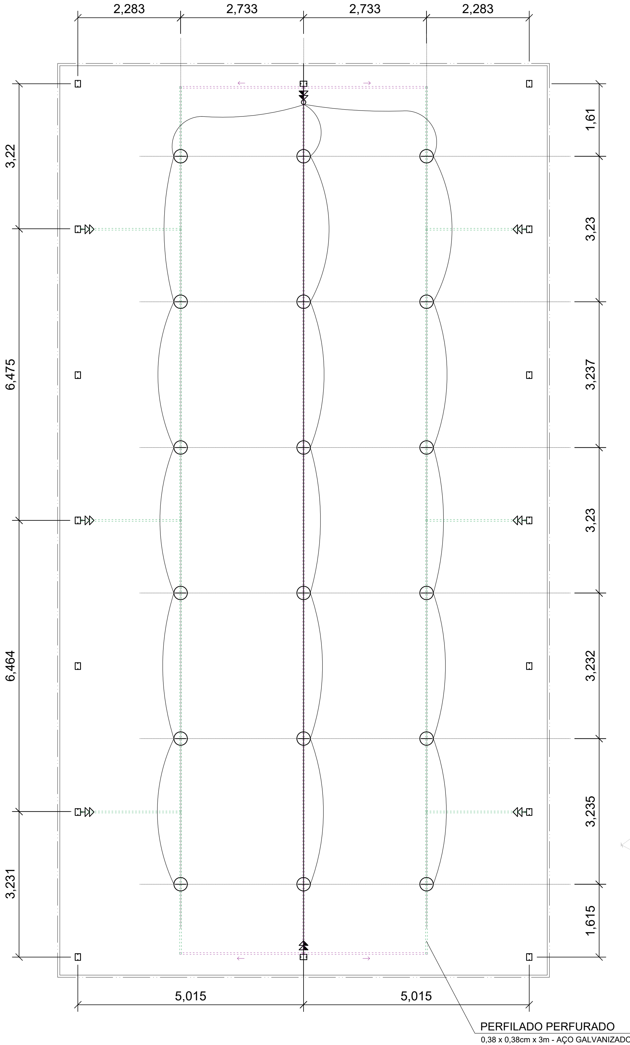
3 ILUMINAÇÃO LAYOUT DE ILUMINAÇÃO E TOMADAS - ESC. 1:75
