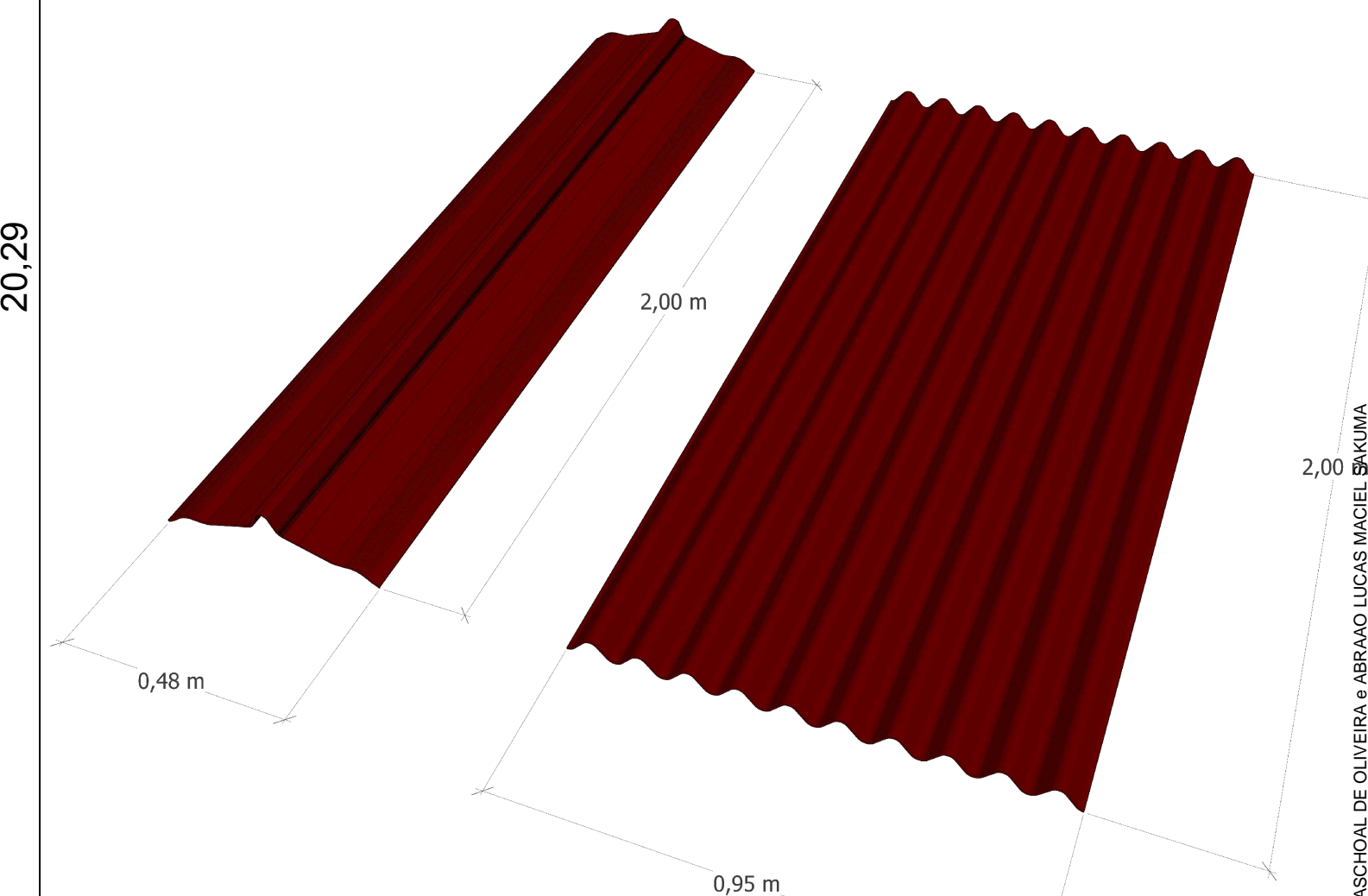
6 ESQUEMA TELHA ECOLÓGICA CUMEEIRA E TELHA - S/ ESC.
