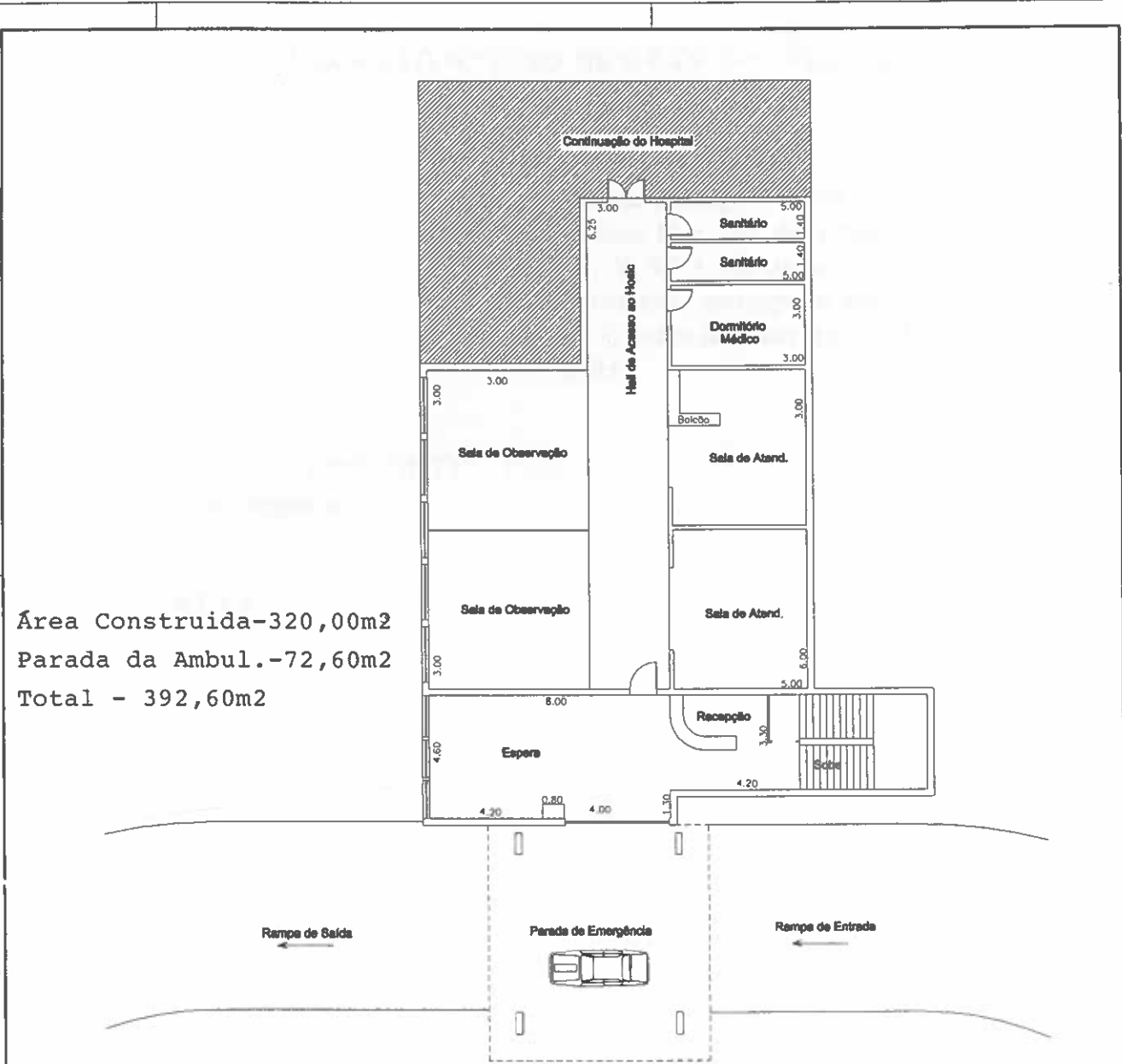
PLANTA BAIXA
