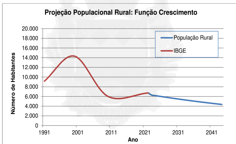
Figura 42: Projeção Populacional Rural: Método da Função Crescimento.
