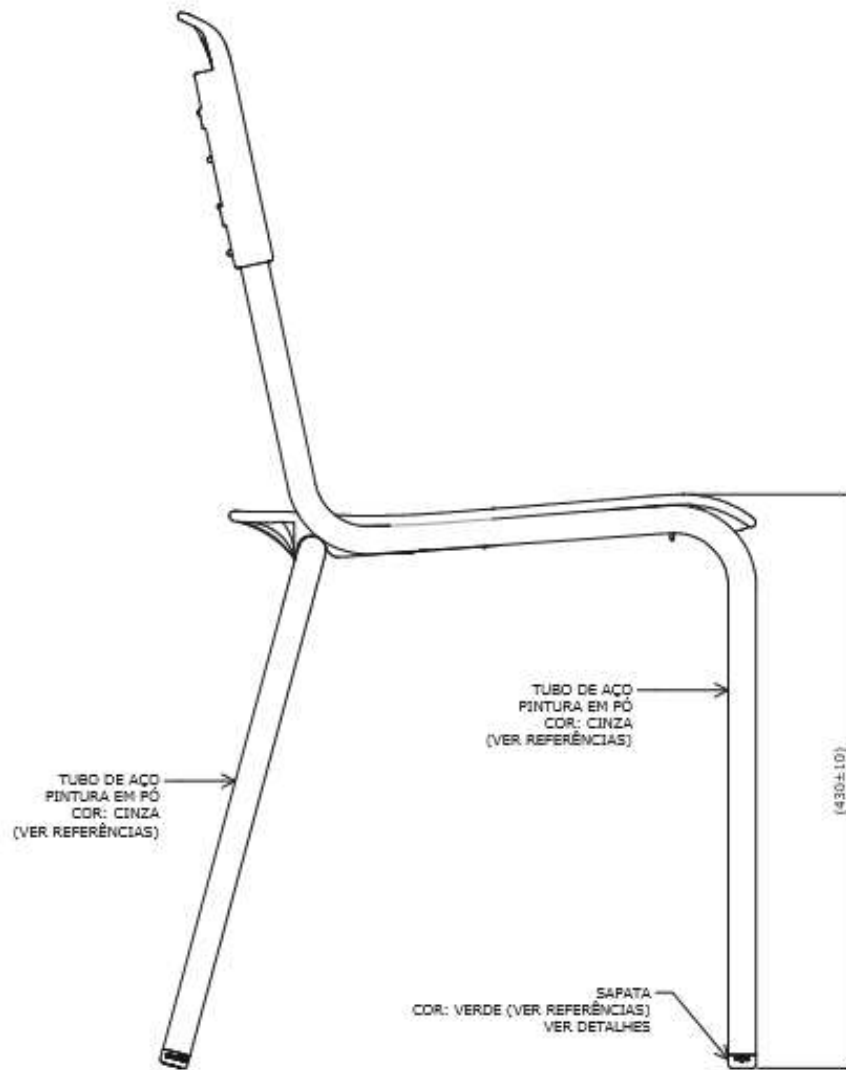
VISTA LATERAL ESC. 1 : 5
