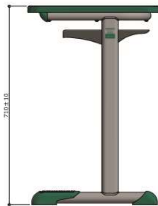
VISTA LATERAL ESC. 1 : 10
