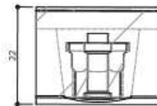
DETALHE G ESC. 1 : 1
