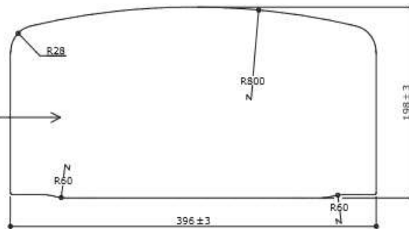
VISTA FRONTAL ESC. 1 : 5
