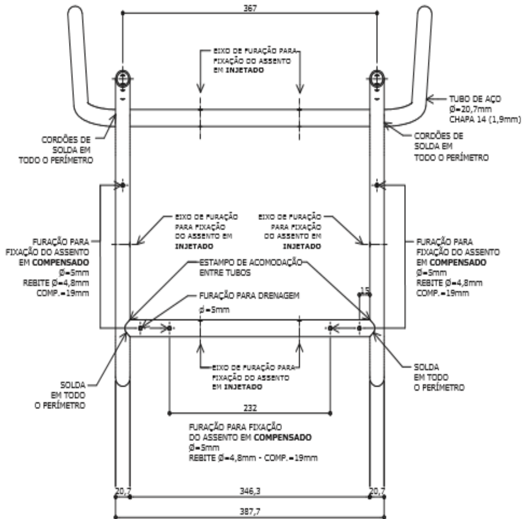
VISTA SUPERIOR DA ESTRUTURA
