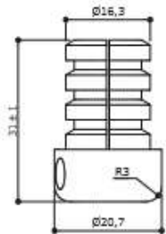
VISTA 2 ESC. 1 : 1
