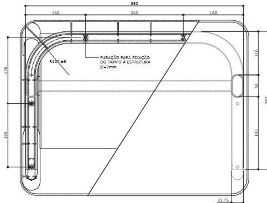
VISTA SUPERIOR ESC. 1 : 5
