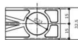
DETALHE D ESC. 1 : 2
