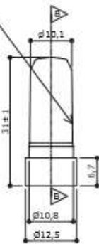
VISTA 3 ESC. 1 : 1
