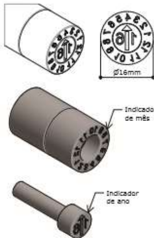
Datador duplo com miolo giratório D= 16mm
