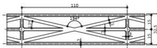
DETALHE C ESC. 1 : 2
