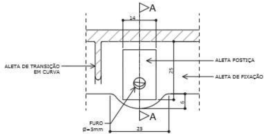
VISTA FRONTAL ESC. 1 : 1
