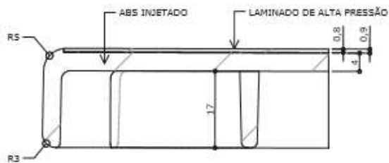
DETALHE F ESC. 1 : 1
