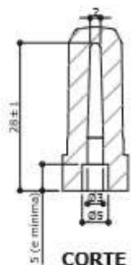
CORTE BB ESC. 1 : 1
