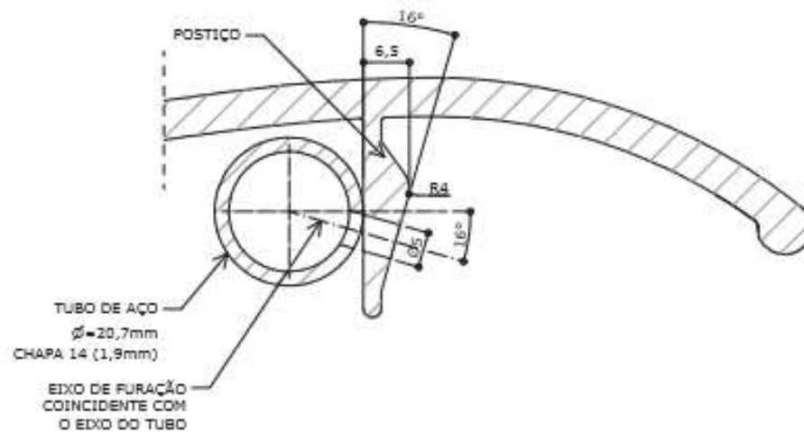
CORTE AA ESC. 1 : 1
