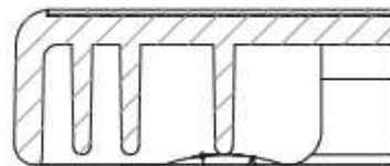
CORTE C-C ESC. 1 : 5
