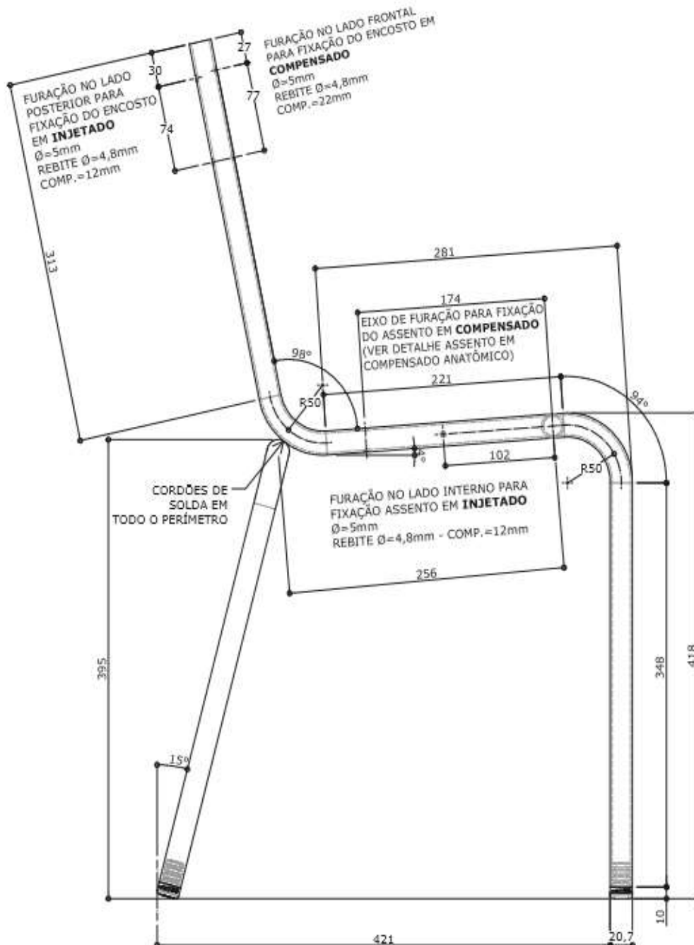
VISTA LATERAL DA ESTRUTURA
