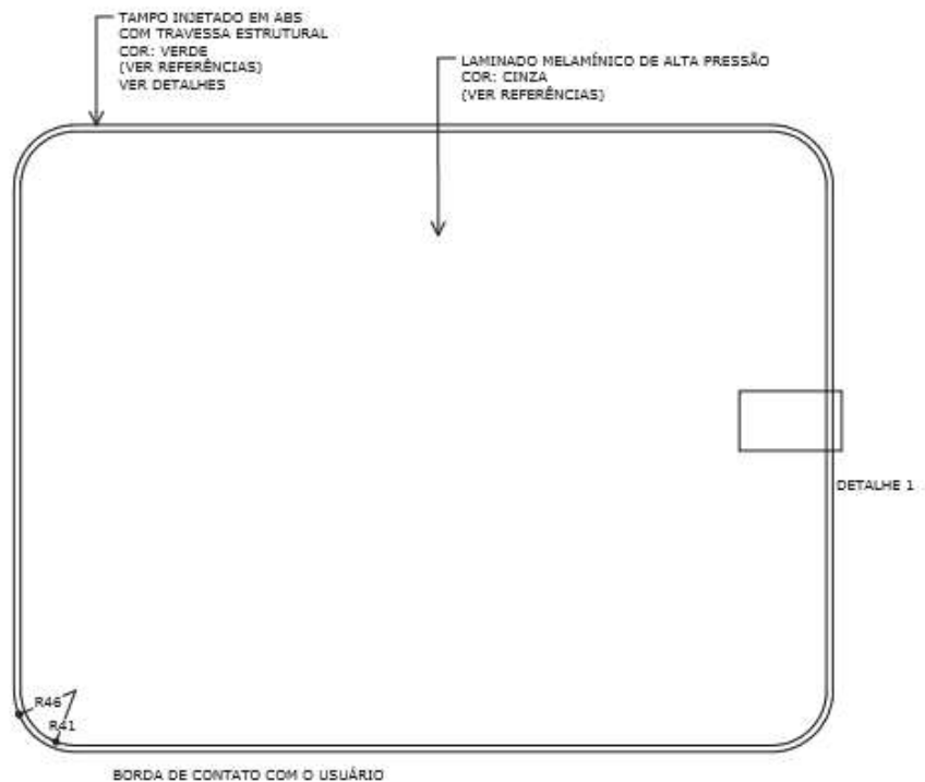
VISTA SUPERIOR - TAMPO ESC. 1 : 5
