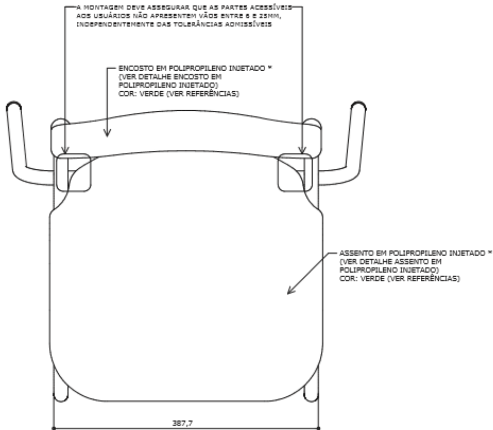
VISTA SUPERIOR ESC. 1 : 5
