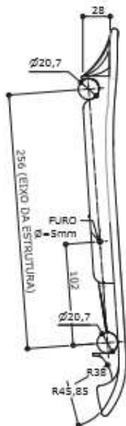
VISTA LATERAL ESC. 1 : 5
