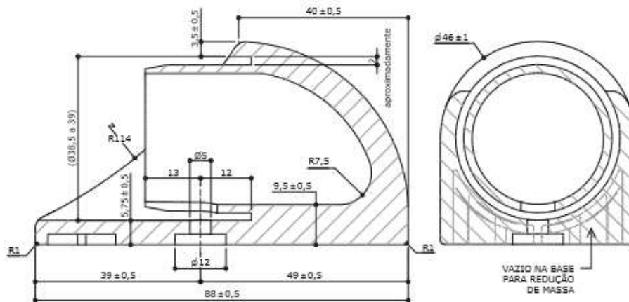
CORTE BB ESC. 1 : 1
