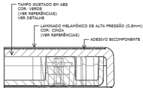
DETALHE 2 ESC. 1 : 1
