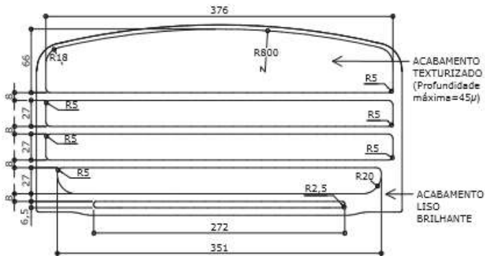
VISTA FRONTAL - ACABAMENTO ESC. 1 : 5
