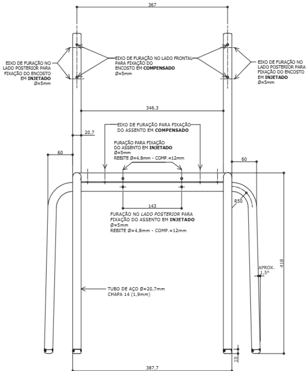
VISTA FRONTAL DA ESTRUTURA
